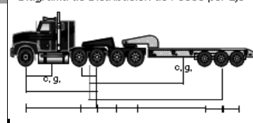
Diagrama de Distribución de Pesos por Eje
